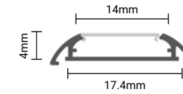
SKU: 5002 Bendable -Silver body (L=1m) ■
